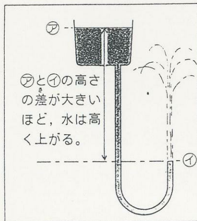
④水がふき上がる原理
